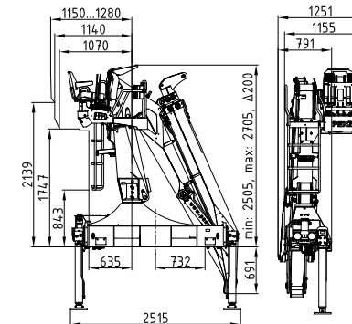
Seitensitz 04 rechts & links Side seat 04 right & left
