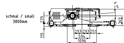
Rücksitz 01 Back seat 01
